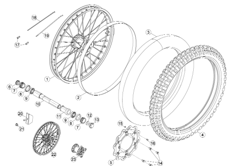
TAV.27 Ruota anteriore - Front wheel - Roue AV. - Vorderrad - Rueda delantera
