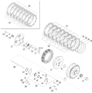
TAV.5 Frizione - Clutch - Embrayage - Kupplung - Embrague
